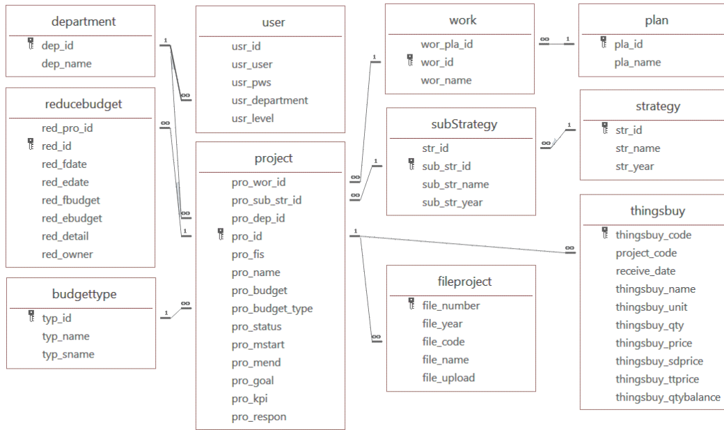
ภาพที่ 3 ความสัมพันธ์ระหว่างตารางข้อมูล (Table Relationship)ระบบบริหารงบประมาณคณะมนุษยศาสตร์และสังคมศาสตร์ มหาวิทยาลัยราชภัฏรำไพวงศ์
