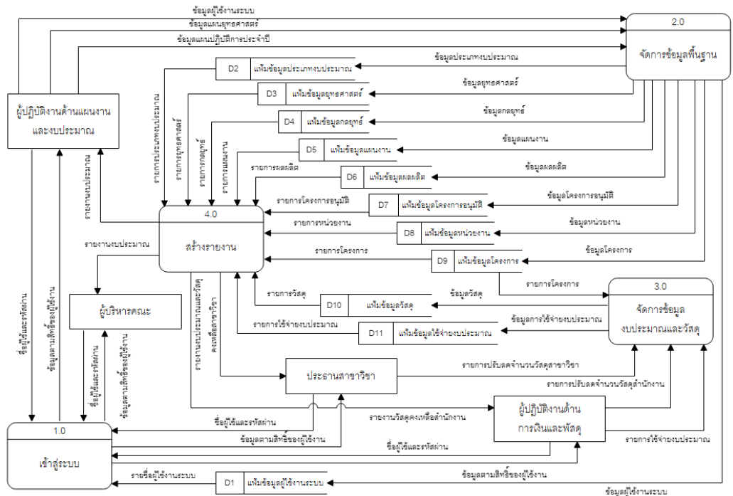
ภาพที่ 2 แผนภาพกระแสข้อมูล (Data Flow Diagram : DFD Level 1) ระบบบริหารงบประมาณคณะมนุษยศาสตร์และสังคมศาสตร์ มหาวิทยาลัยราชภัฏลำปาง
