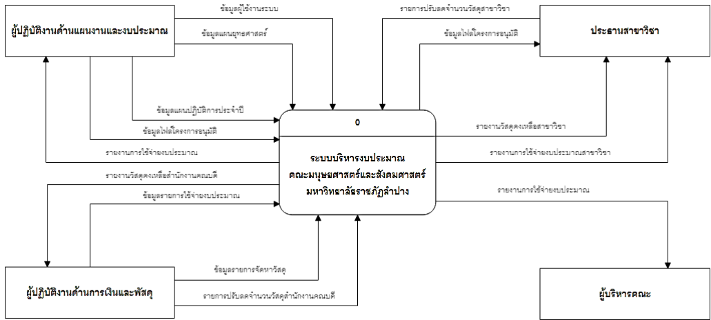
ภาพที่ 1 แผนภาพกระแสข้อมูล (Data Flow Diagram : DFD Level 0)ระบบบริหารงบประมาณคณะมนุษยศาสตร์และสังคมศาสตร์ มหาวิทยาลัยราชภัฏลำปาง
